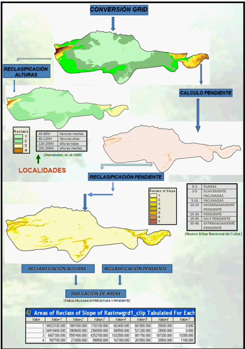
Figura 4 – Obtención de los mapas de los pisos altitudinales e inclinación de la pendiente reclasificados
