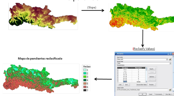
Figura 4 – Obtención y reclasificación del mapa de pendientes a partir del MDE
