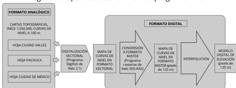
Figura 2 – Modelo digital de elevación del estado de Hidalgo. Pasos generales para su obtención con el programa Ilwis
